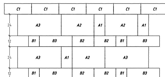
Muro H=72cm posa a "Correre" (2/3 tipo "A" - 1/3 tipo "B")
