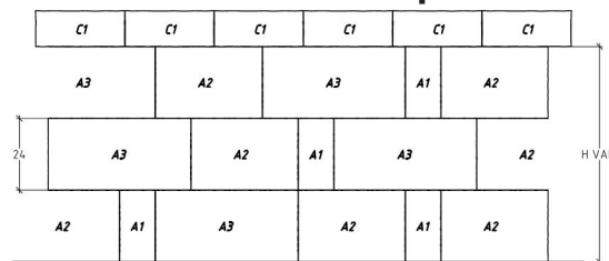
Muro H=72cm posa a "Corsi regolari" (solo tipo "A" o tipo "B")
