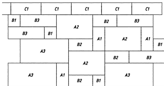
Muro H=72cm posa alla "Romanica" (2/3 tipo "A" - 1/3 tipo "B")
